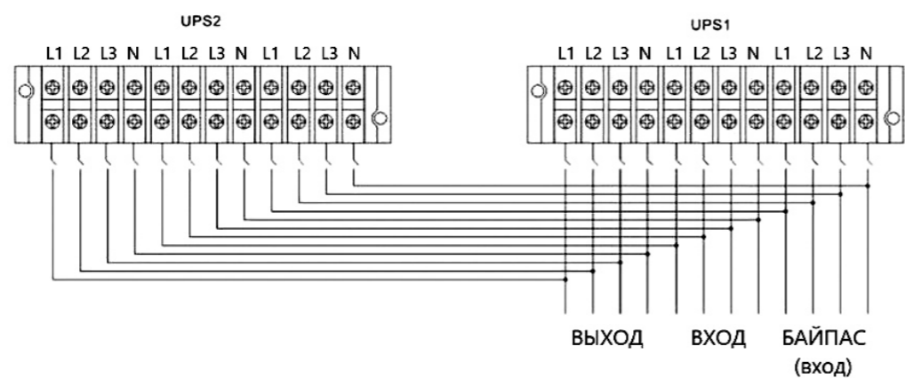
Монтажная схема параллельной системы для 15000 DUAL
