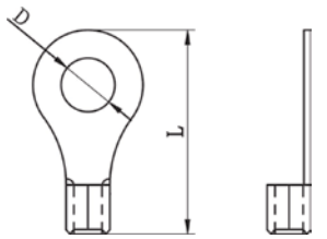
Кольцевой наконечник
